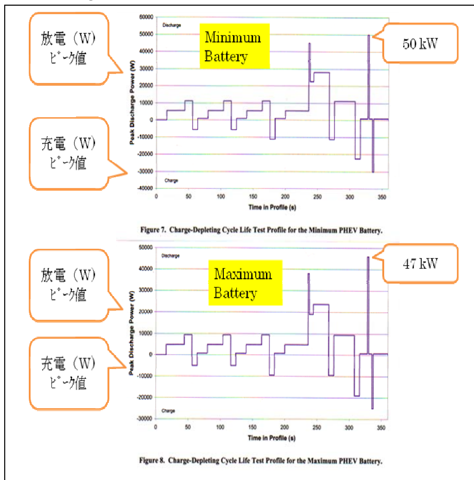
図 5-11 (Figure-7, 8) 枯渇/CD モードにおけるサイクル寿命試験のプロファイル
