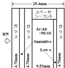
図72 Suntuitive™の断面構造
