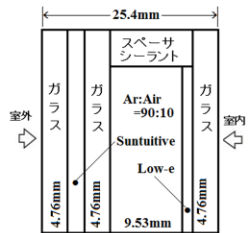
図72 SuntuitiveTMの断面構造
